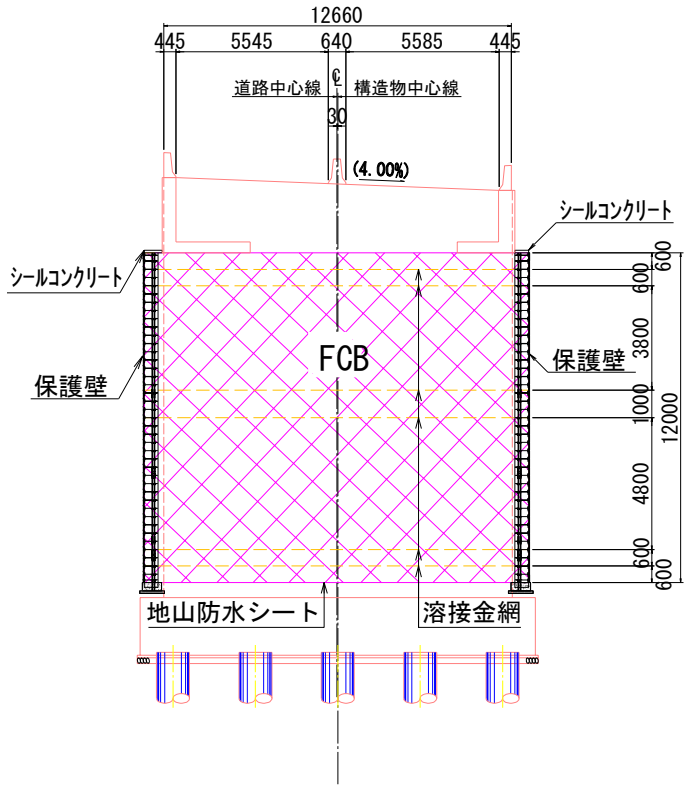
FCB横断面図 S=1:100 (C-C断面)
