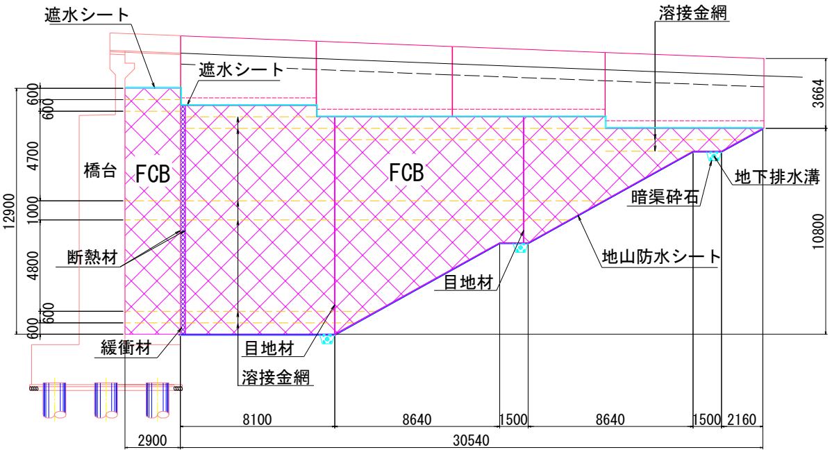
FCB側面図 S=1:100 (B-B断面)
