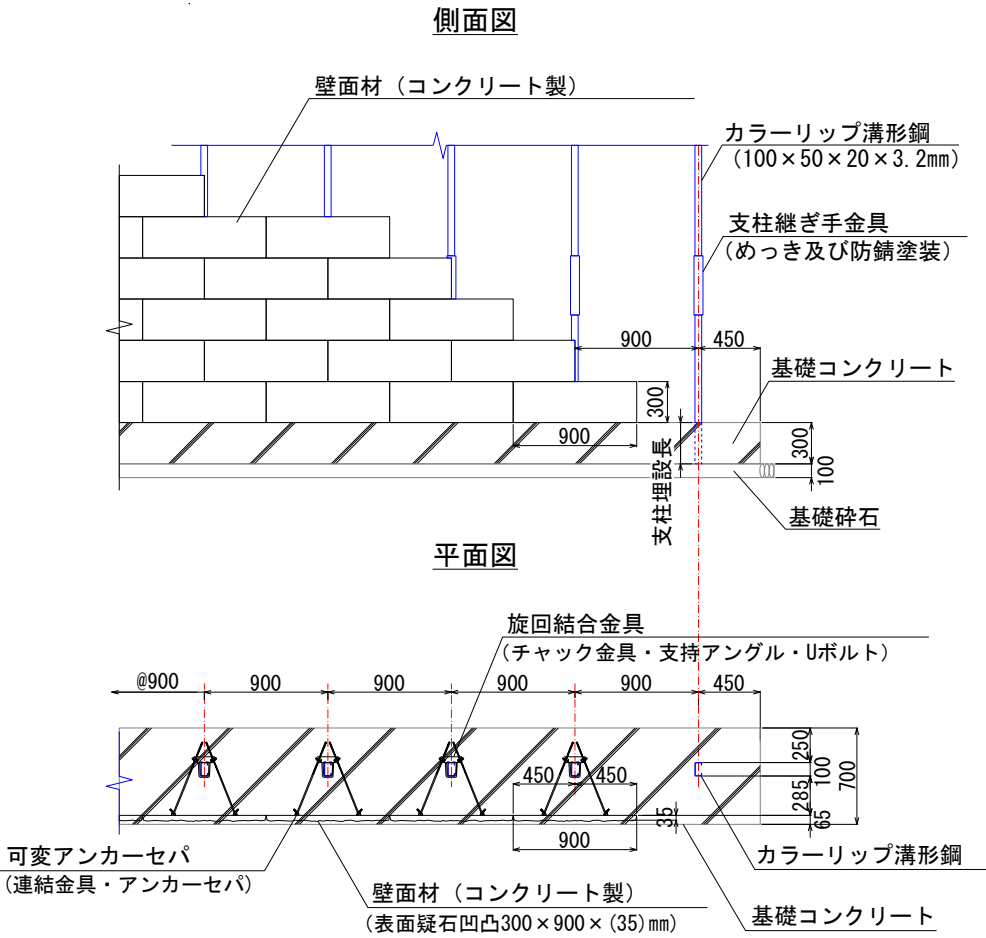
3FCB保護壁設置工 標準図 S=1:20
