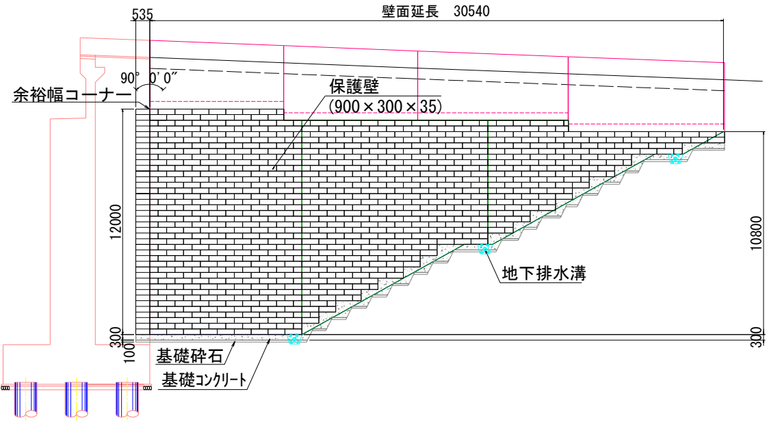
FCB壁面展開図 S=1:100 (A-A断面)
